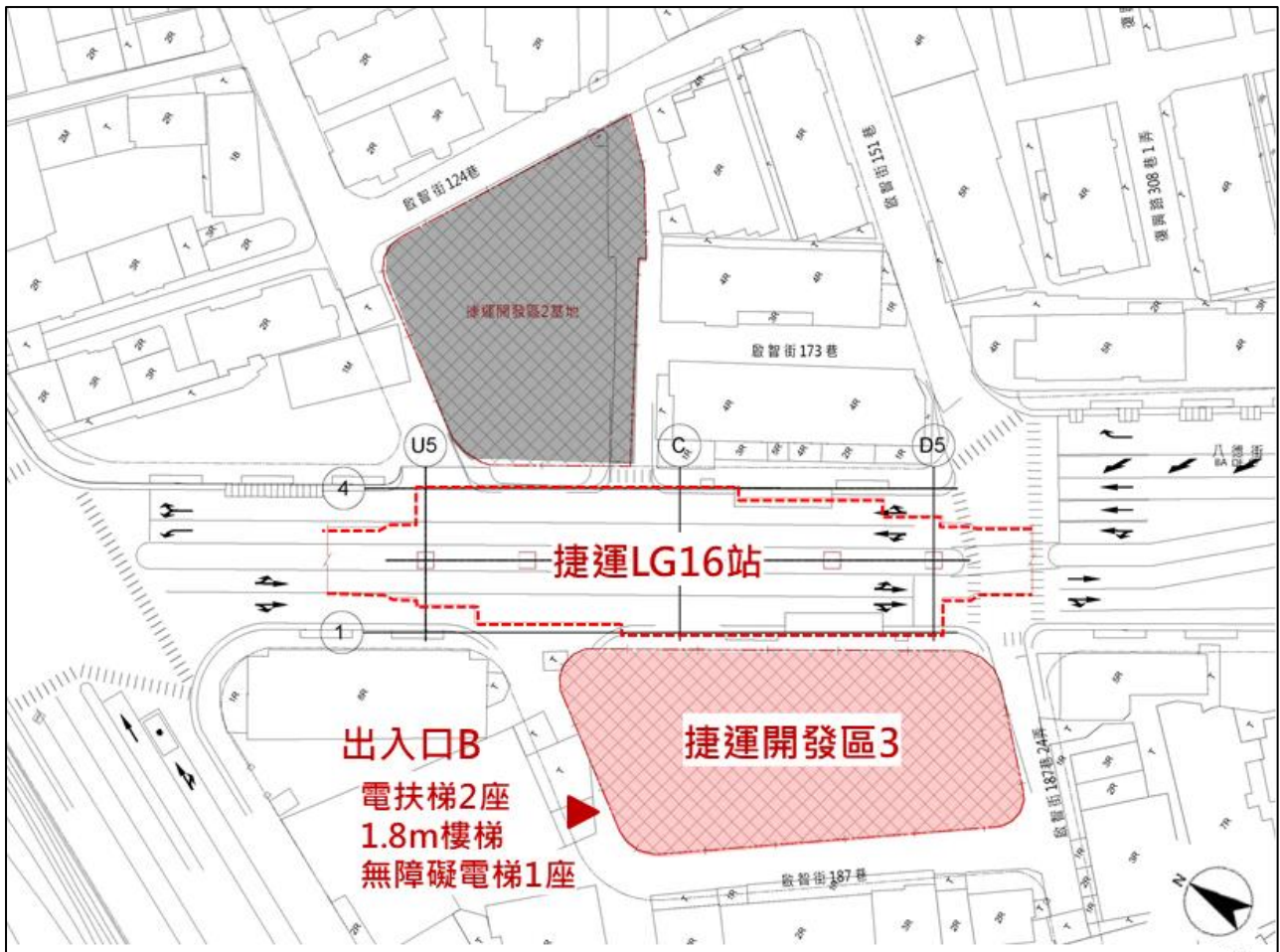
圖三 捷運出入口位置圖
