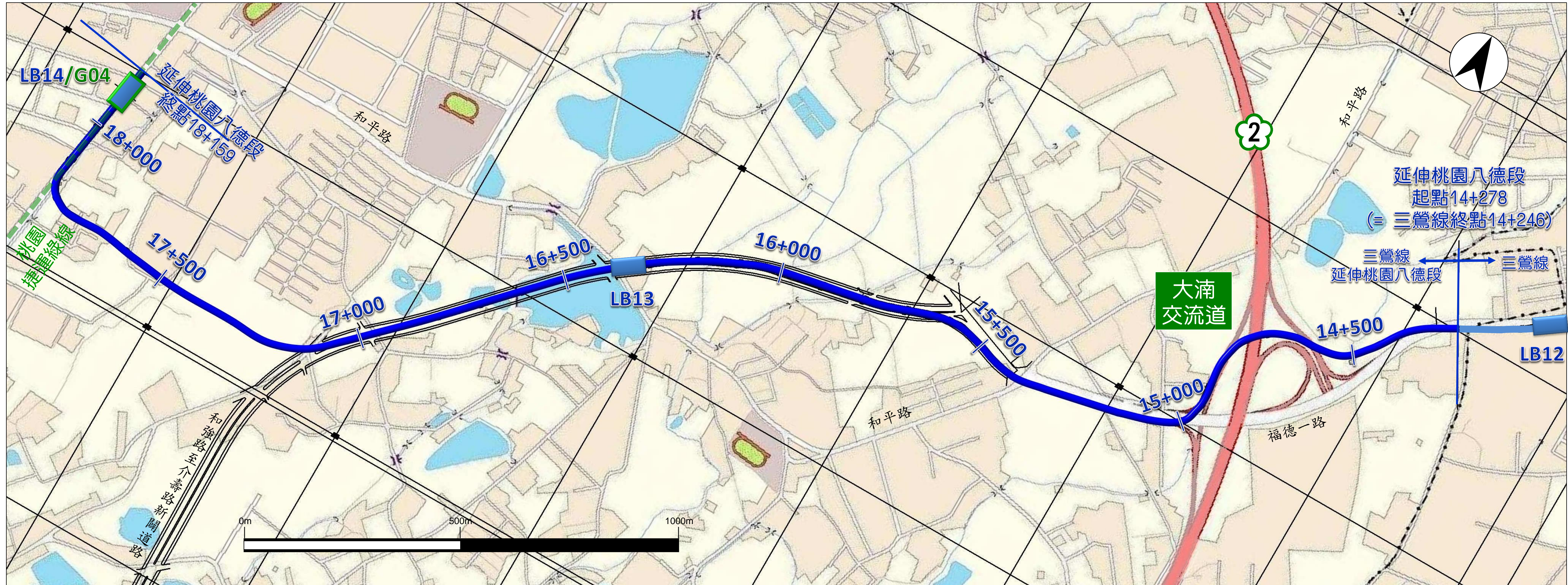
圖9.2-2 捷運三鶯線延伸桃園八德段路線平面圖 (比例尺1/5,000)
